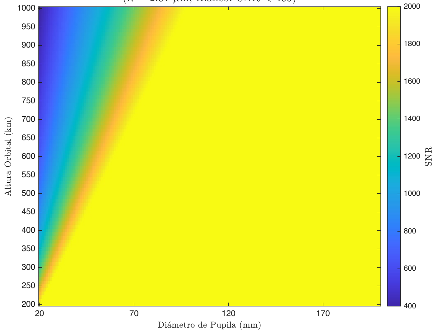
SNR - Refractivo - Detector 3 ( \lambda = 2.01 \mu\text{m} , Blanco: SNR < 400)
